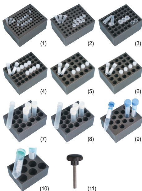
Bloque calefactor "MaXtable™ H2O"
